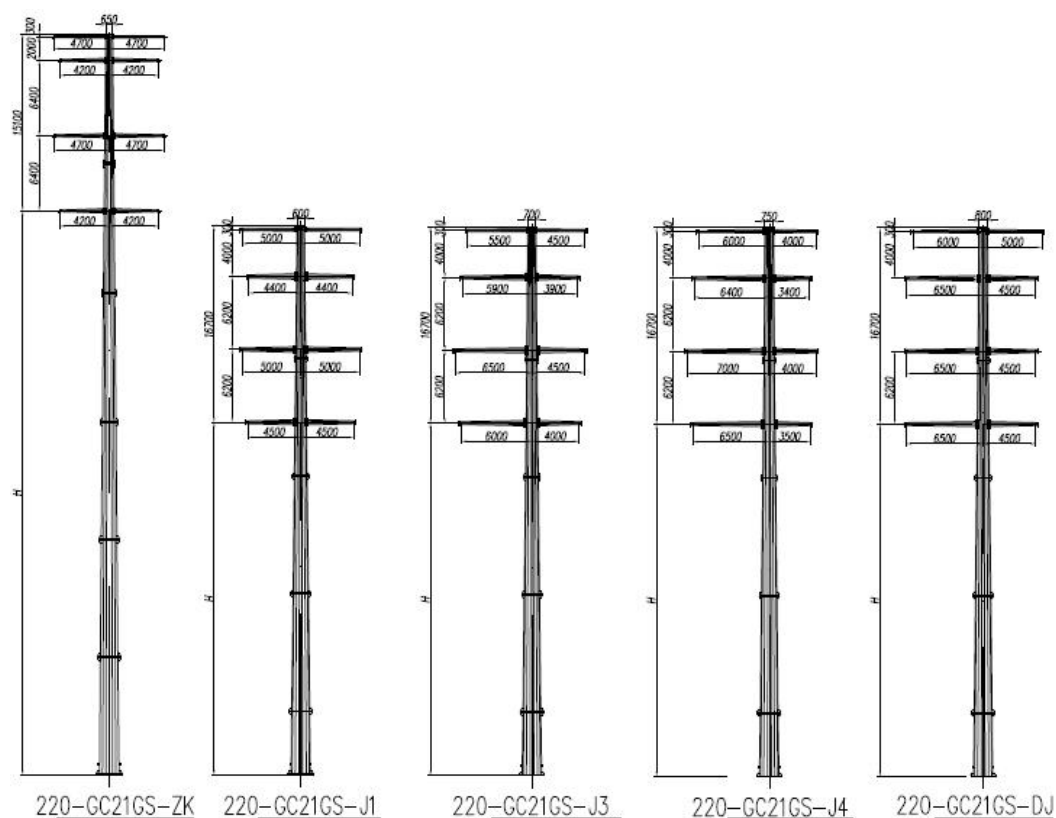
图 1.1-3 塔基型号图
