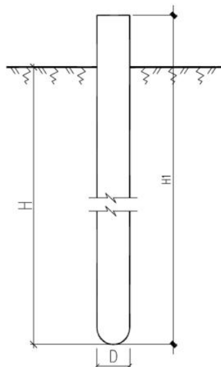
图 1.1-2 塔基基础示意图
