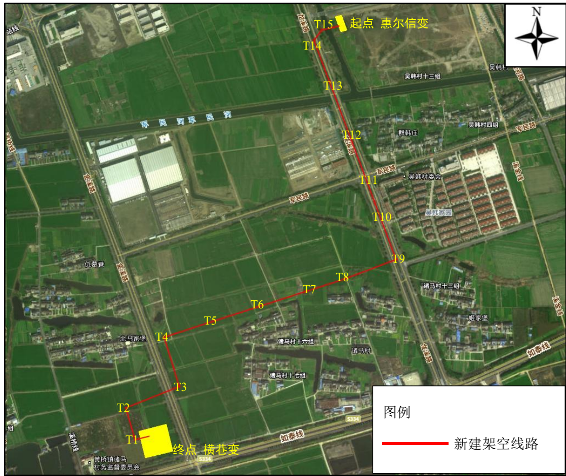
图 1.1-1 线路路径示意图
