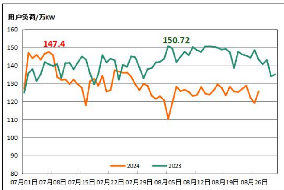
图 5-2 110kV 及以上大用户最高负荷曲线
