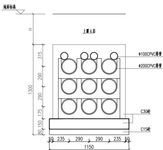
图 1.1-6 双回电缆排管断面图
