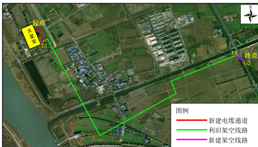
图 1.1-2 天星~七圩、天星~双越 110 千伏线路路径示意图
