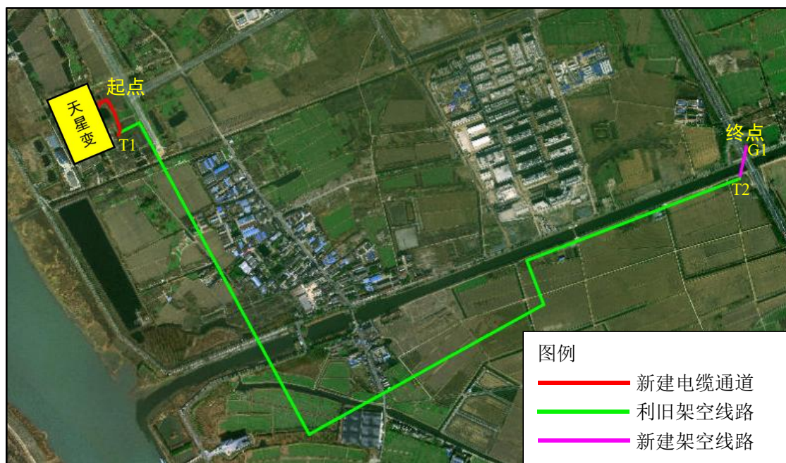
图 1.1-1 天星～朝阳、天星～洋思 110 千伏线路路径示意图
