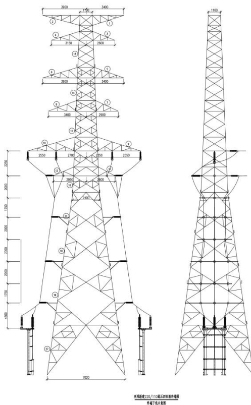
图 1.1-5 电缆引下平台示意图
