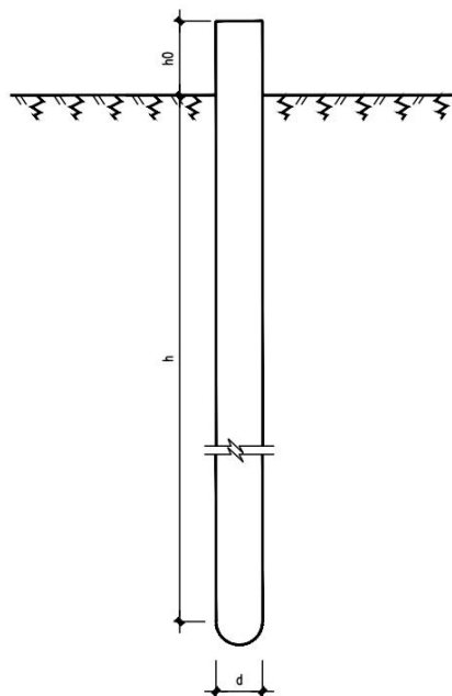
单桩灌注桩基础(B)
