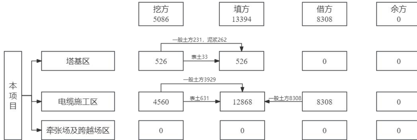
图 1.1-18 工程总土石方平衡流向框图 单位: m 3
