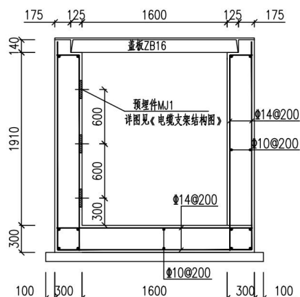
图 1.1-7 工井断面图
