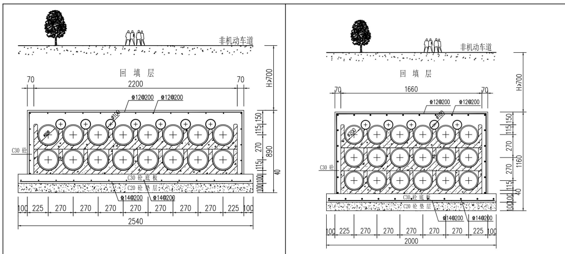
图 1.1-7 2×8Φ200+7Φ100 排管（普通型）
