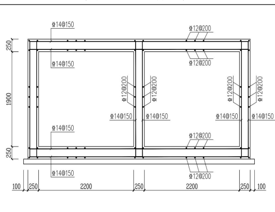
图 1.1-6 进站双拼电缆井土建断面图
