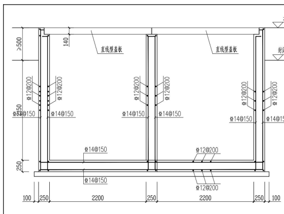
图 1.1-5 双拼直线井土建断面图
