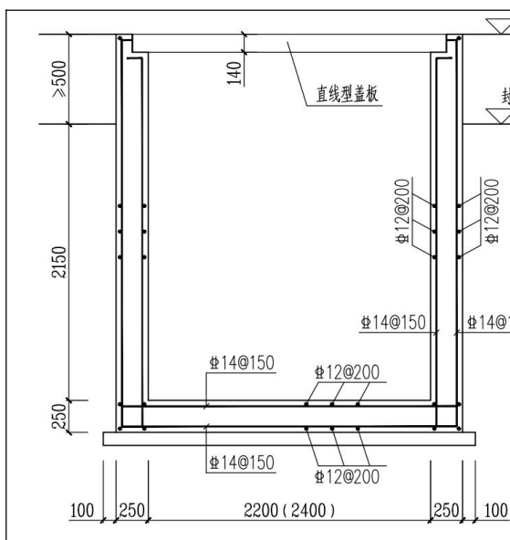
图 1.1-3 三通井、进站电缆井土建断面图
