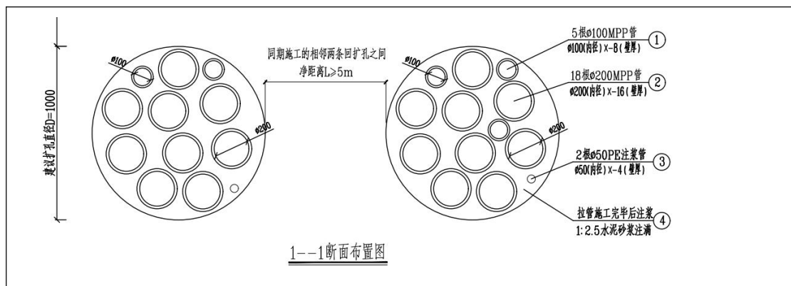
图 1.1-12 18Φ200+5Φ100 拉管土建断面图
