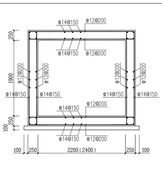
图 1.1-4 1#直线井、2#直线井、中间接头井、转角井土建断面图
