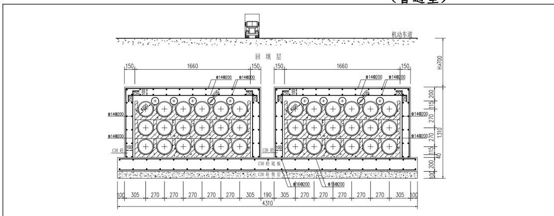
图 1.1-11 2×3×6Φ200+2×5Φ100 排管（加固型）土建断面图
