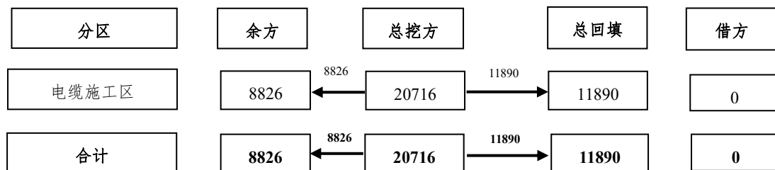
图 1.1-13 土石方平衡流向框图 单位: m 3
