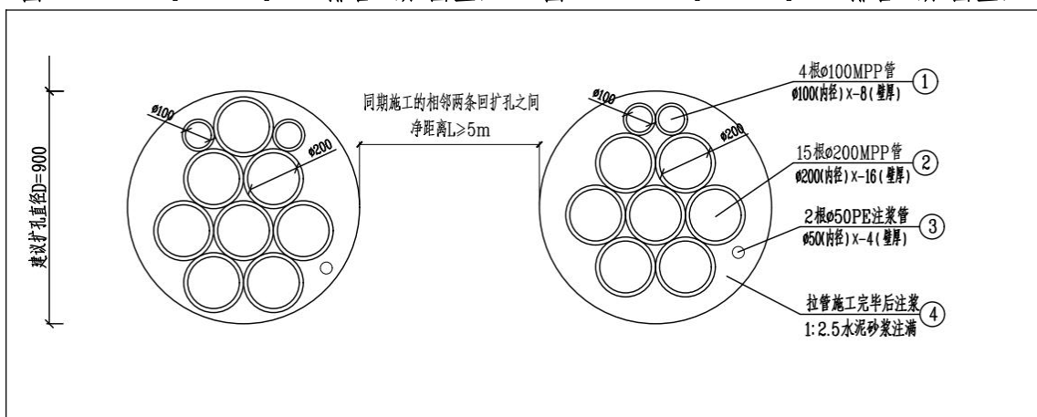
图 1.1-10 15 φ200+4 φ100 拉管
