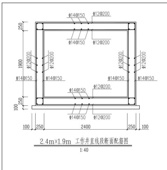
图 1.1-6 三通井土建断面图
