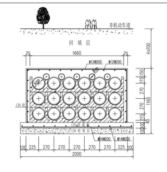
图 1.1-7 3×6 φ200+5 φ100 排管 (普通型)
