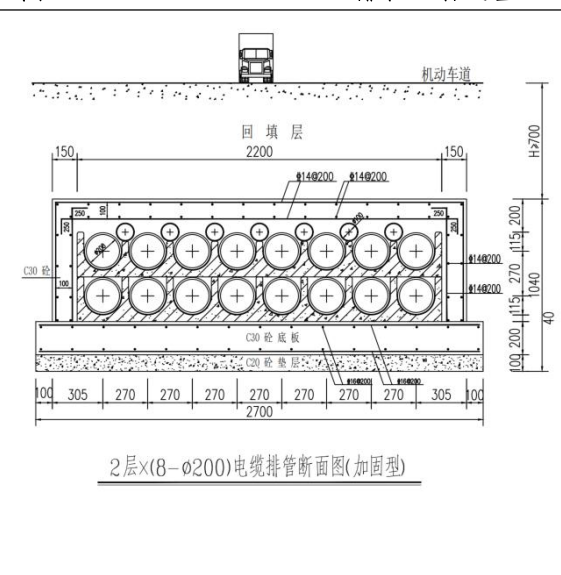
图 1.1-9 2×8 φ200+7 φ100 排管 (加固型)
