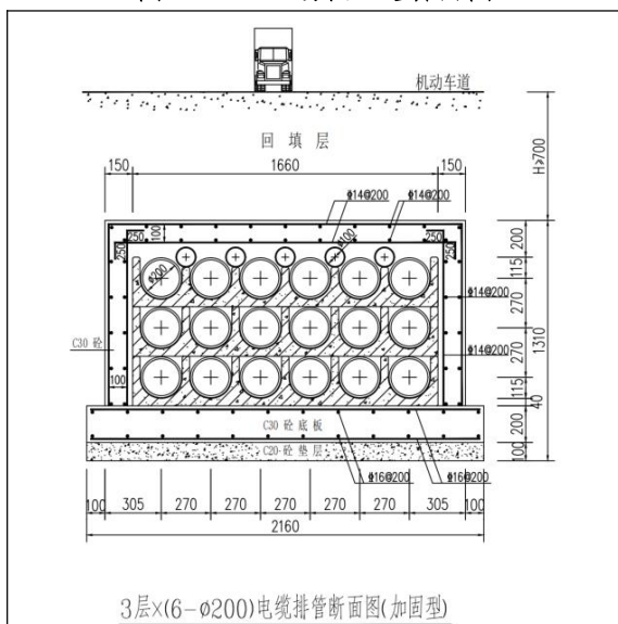
图 1.1-8 3×6 φ200+5 φ100 排管 (加固型)
