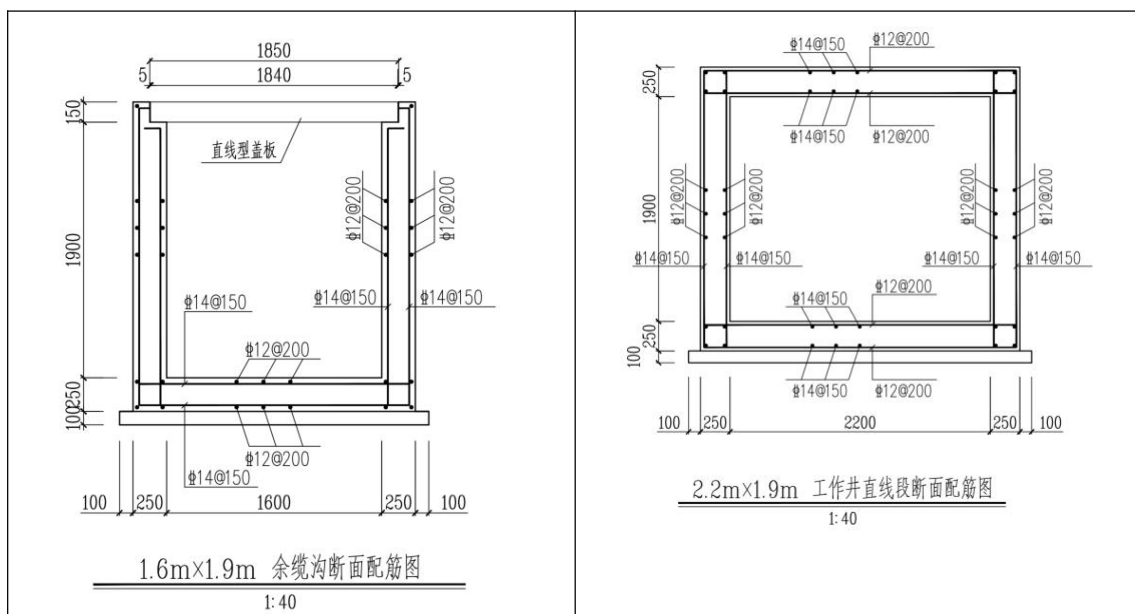
图 1.1-4 余缆沟土建断面图
