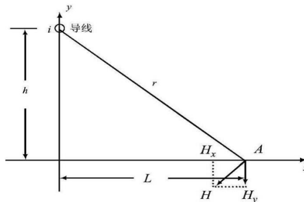
图 3.2-4 磁场向量图
