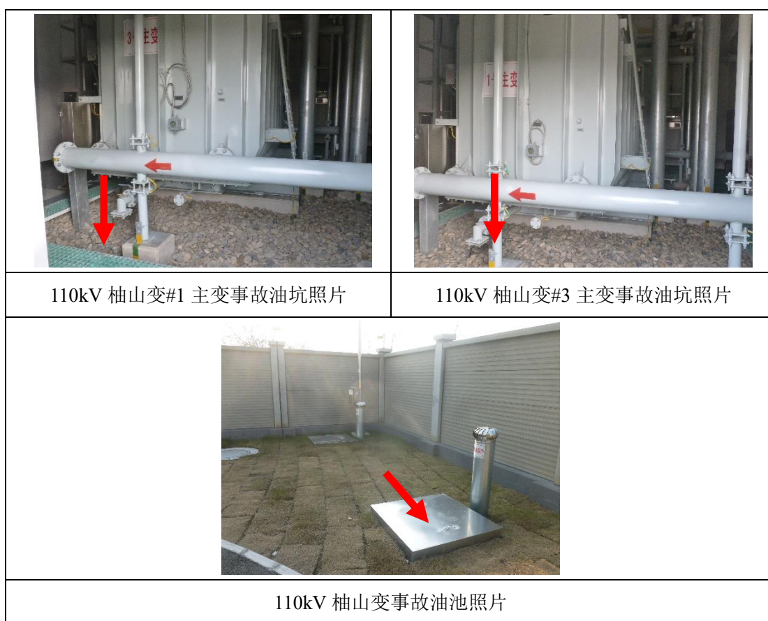
图 8-4 本项目 110kV 柚山变事故油坑及事故油池照片
