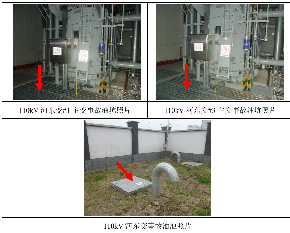
图 8-4 本项目 110kV 河东变事故油坑及事故油池照片
