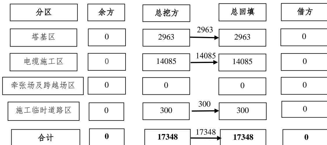
图2-2 土石方平衡流向框图 单位：m 3
