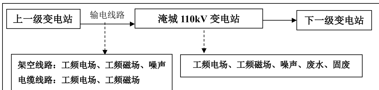
图 2 江苏常州淹城 110kV 输变电工程工艺流程及产污环节示意图
