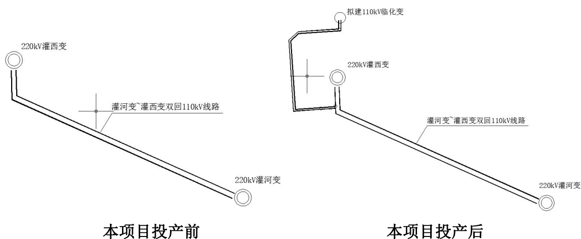
图 2-1 投产前后电网接线示意图
