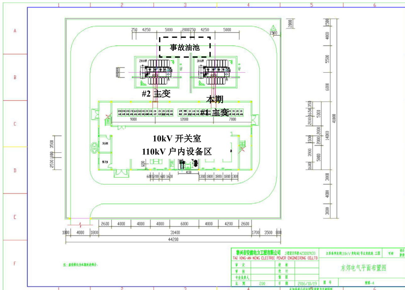
附图3 110kV 东郊变电站平面布置示意图
