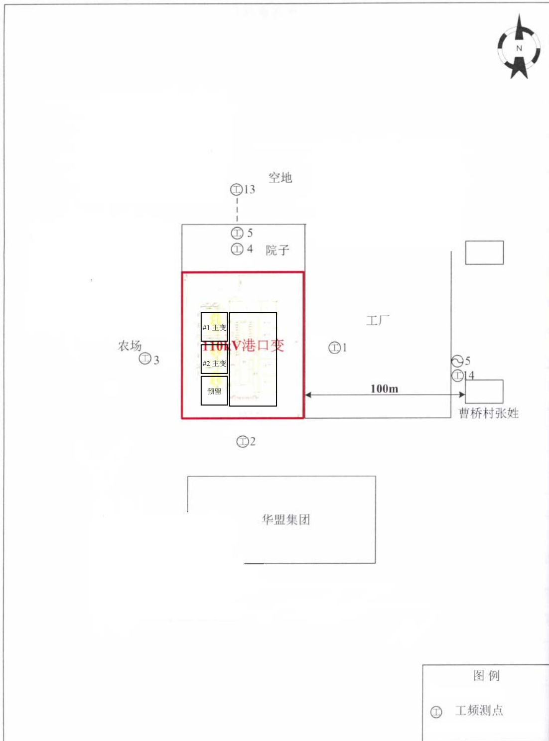
附图4 110kV港口变电站（类比站）监测点位示意图
