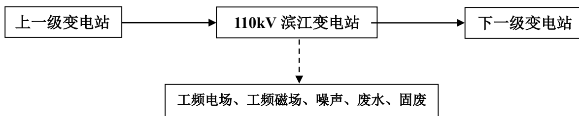
图 1 110kV 主变改造工程工艺流程及产污环节示意图
