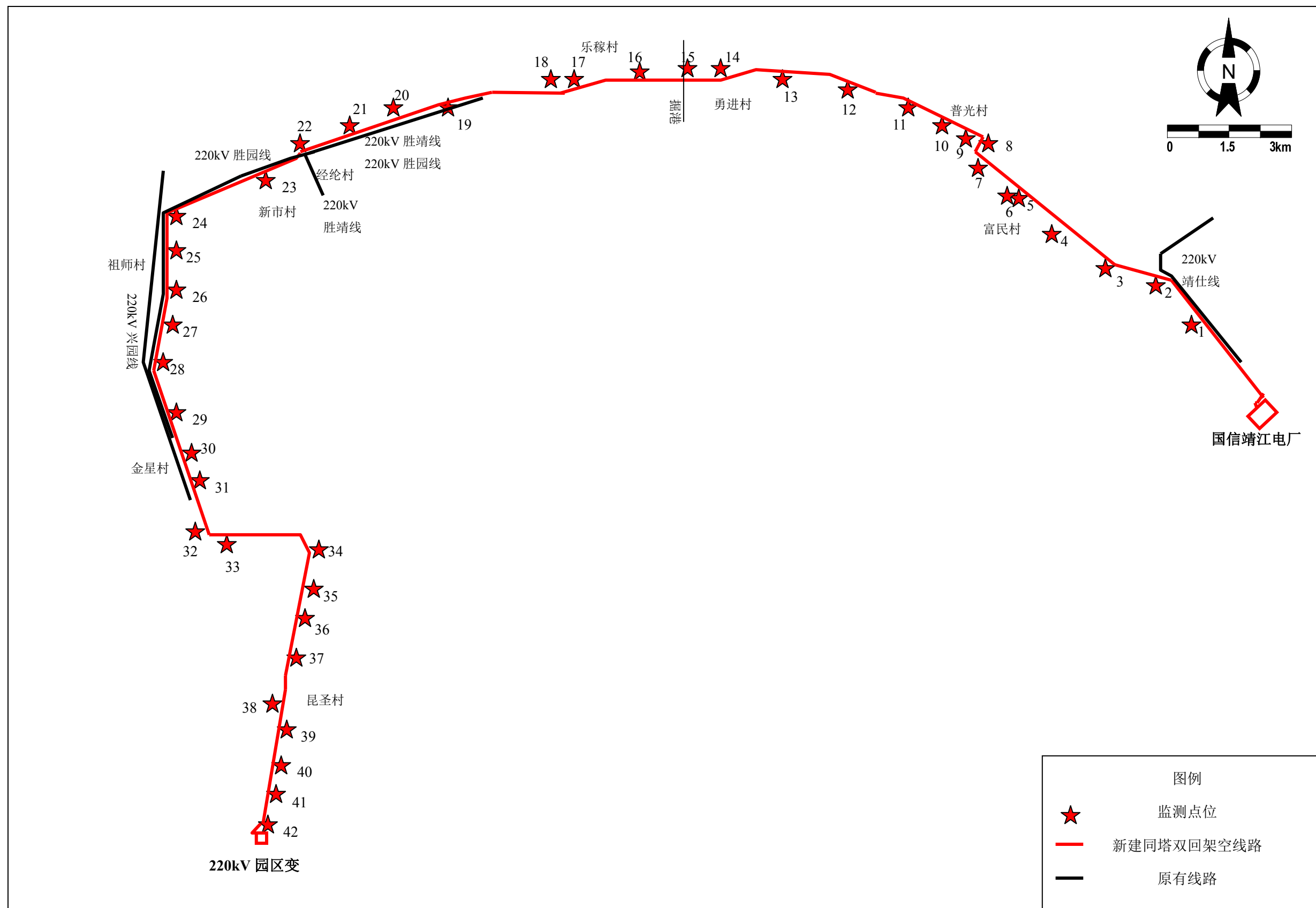
附图 2 国信靖江电厂 2#机组 220kV 送出工程线路路径及监测点位示意图
